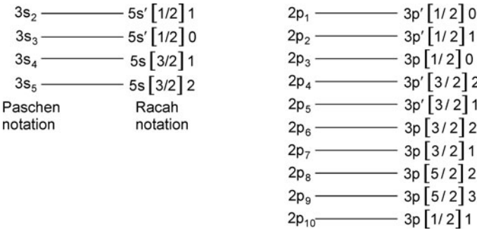
Fig. 14.4 Sublevels of Ne
